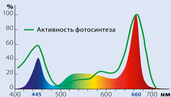
Спектр свечения
