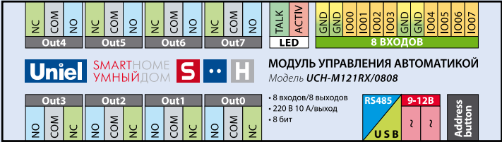
ВЫХОДЫ УПРАВЛЯЮЩИХ РЕЛЕ для ПОДКЛЮЧЕНИЯ ЭЛЕКТРОПРИБОРОВ
