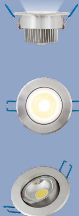
Поворотный механизм
